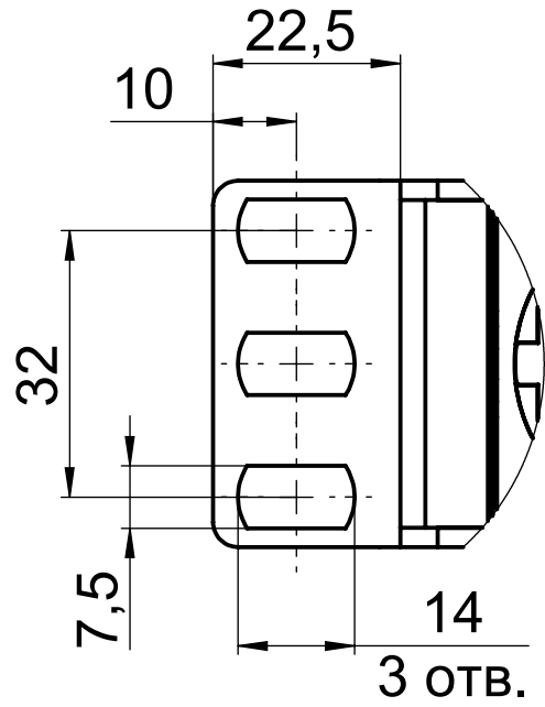
A (1 : 1)
